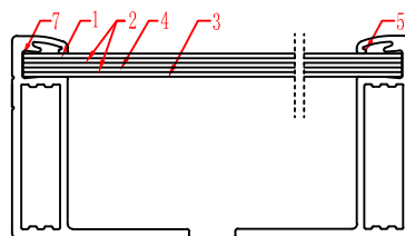
A-A 处放大图 10:1
