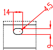
B处放大图 5:1
